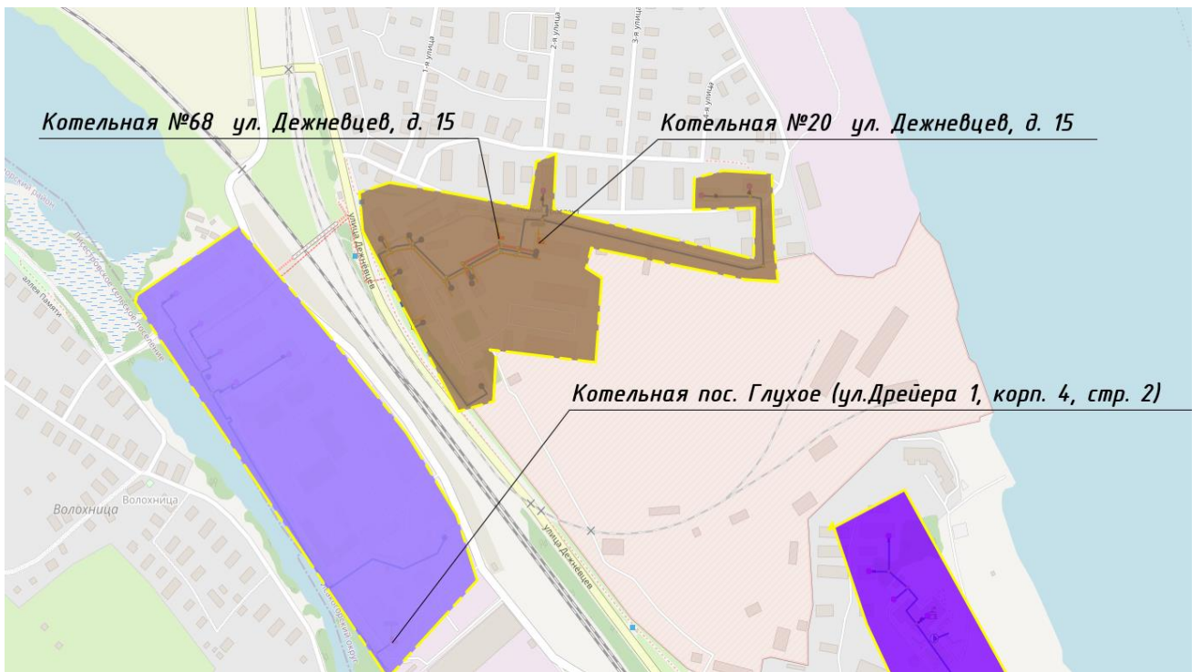
Рисунок 4. Зоны действия котельных ФГБУ «ЦЖКУ» МО России и Котельной п. Глухое (ул. Дрейера 1, корп. 4, стр. 2)
