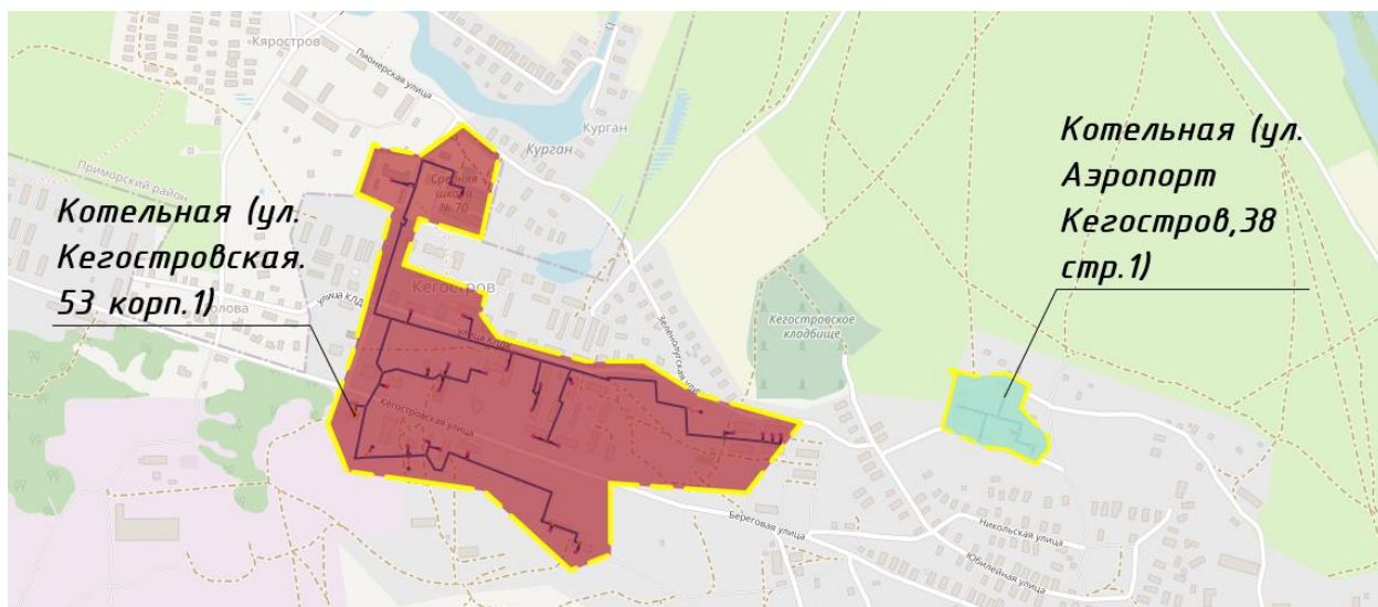
Рисунок 10. Зоны действия котельных ул. Кегостровская 53, корп. 1 и ул. Аэропорт Кегостров 38, стр. 1
