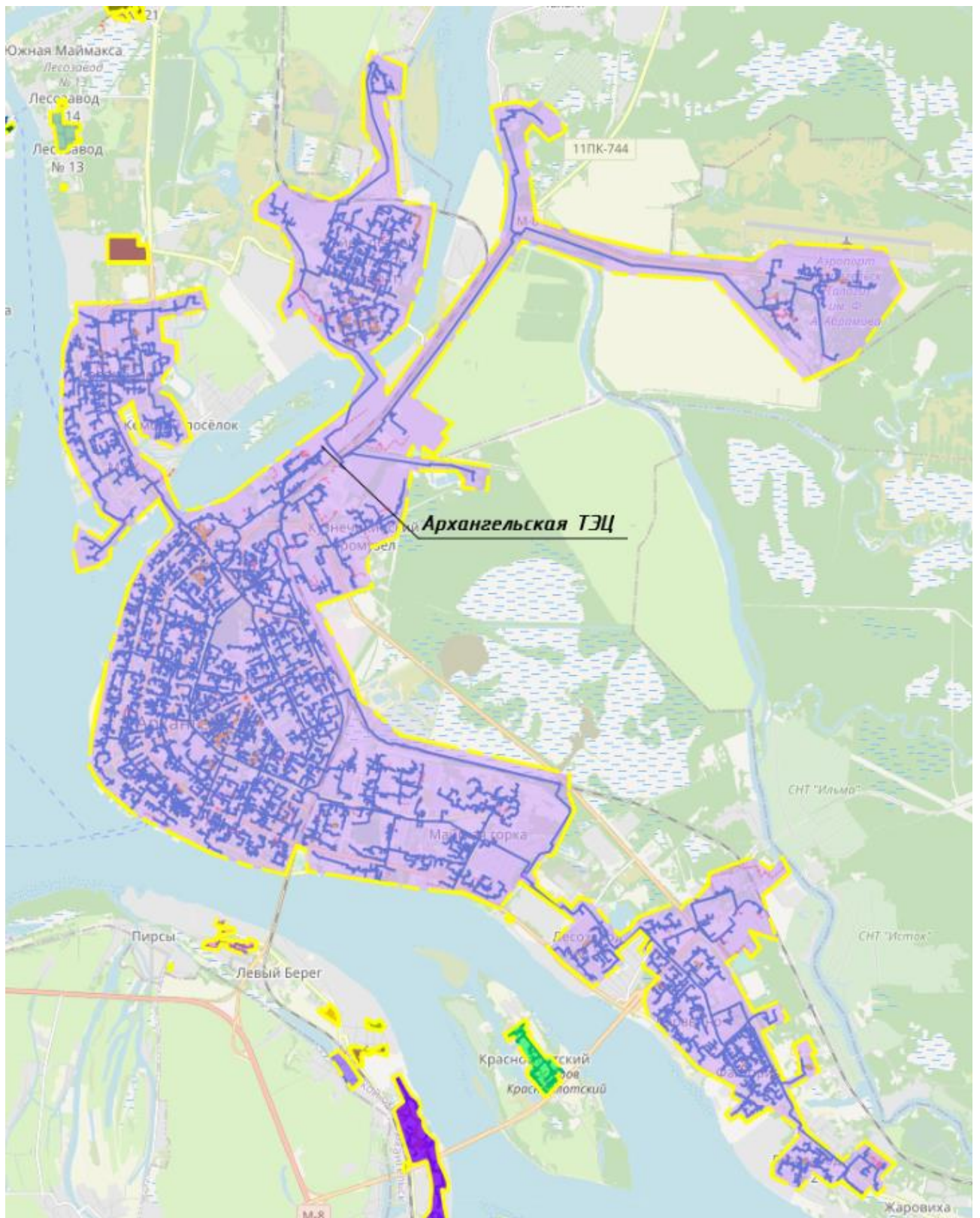
Рисунок 1. Зона действия Архангельской ТЭЦ
